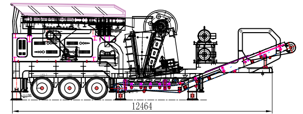
1142 75 鄂破车
