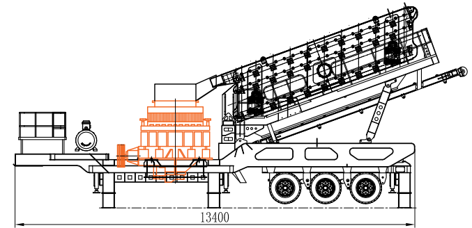
CS160 3-2160圆锥车
